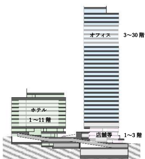
▲断面図
